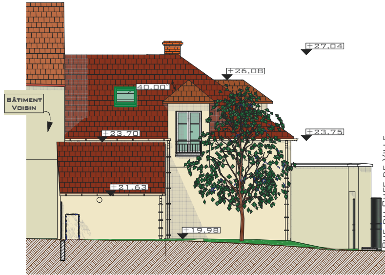
FAÇADE EST SUR JARDIN
