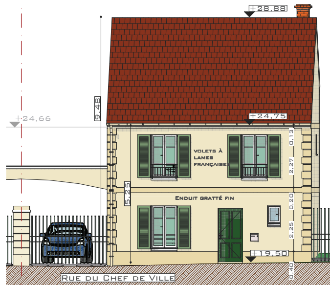
FAÇADE NORD SUR RUE
