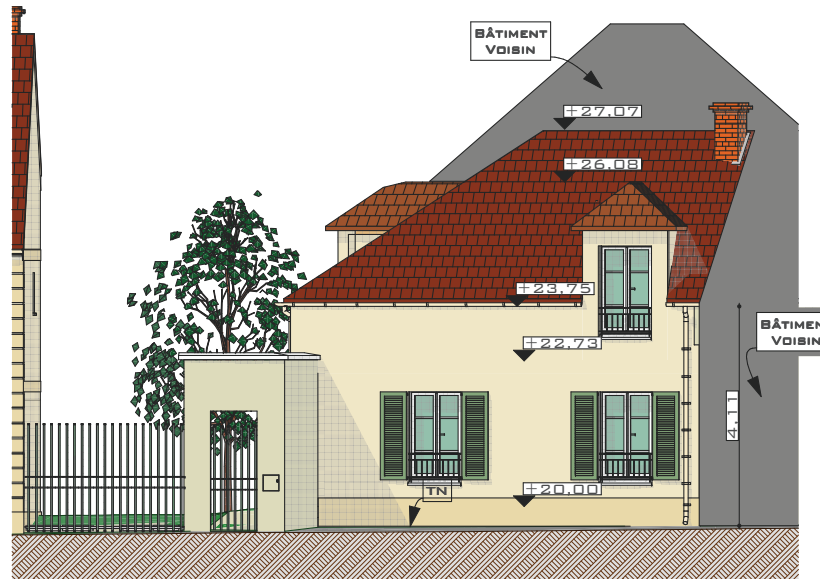
FAÇADE NORD SUR RUE
